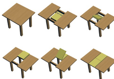
Механизм «Люкс»
