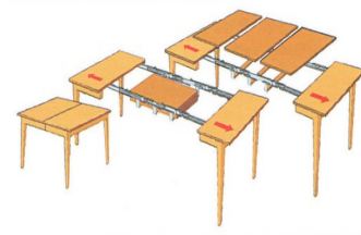
Механизм «Сигма»
